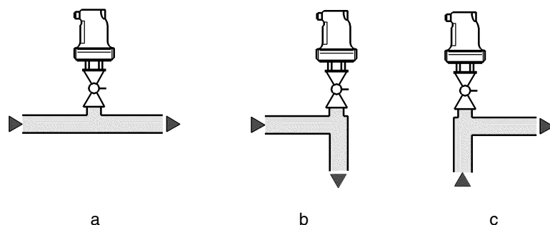
Figure 11 — Emplacement des purgeurs d'air
