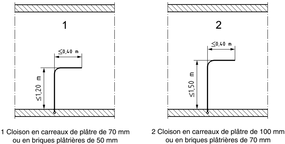
Figure 10 — Tracé des saignées — Elévation
