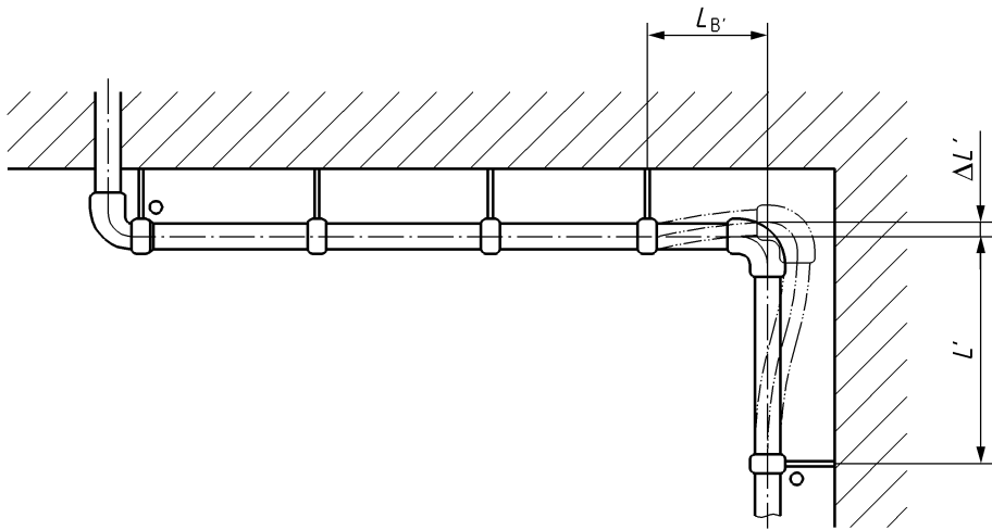
Figure B.1 — Dilatation d'un bras flexible
